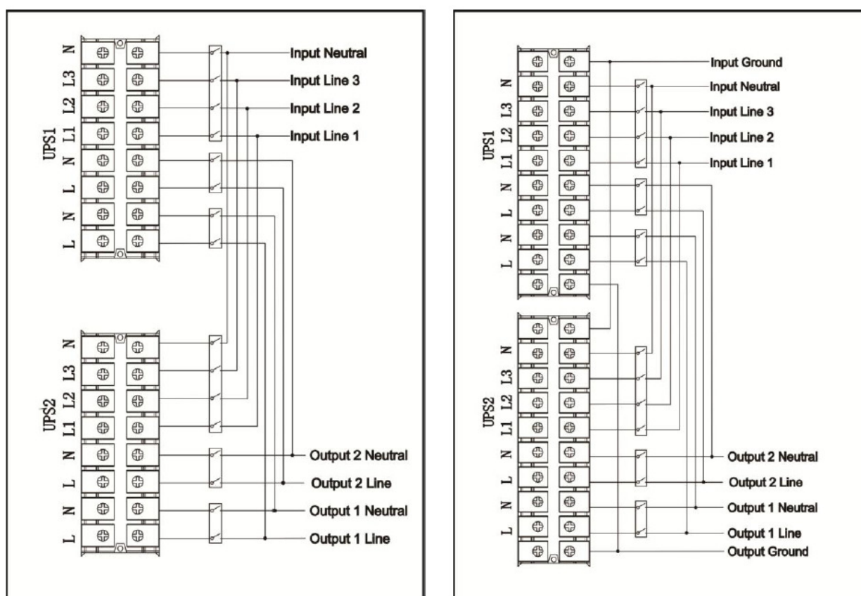
Figura 7 - Collegamenti del Sistema Parallelo
